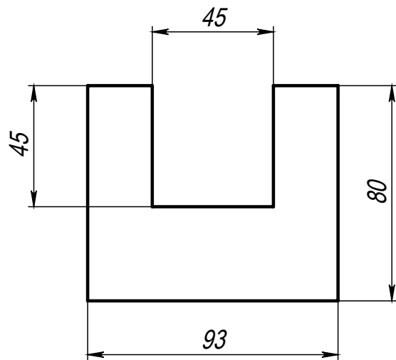
Поз.2 (Ребро)
